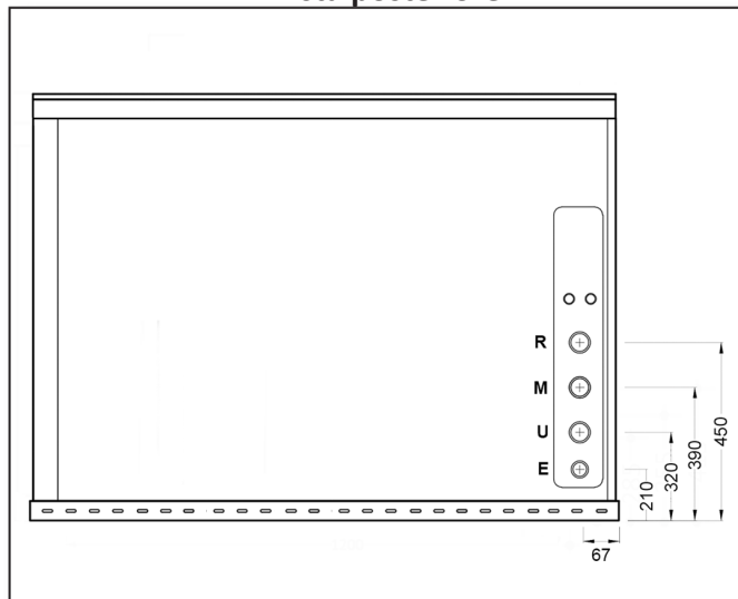
Vista posteriore
