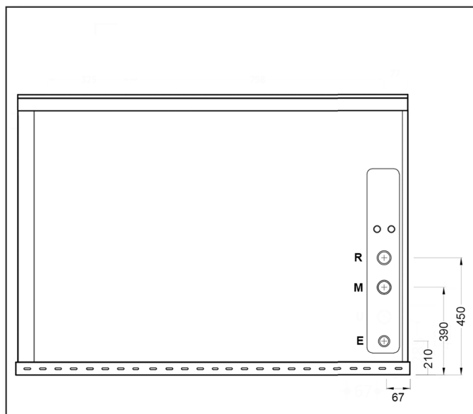
Vista posteriore
