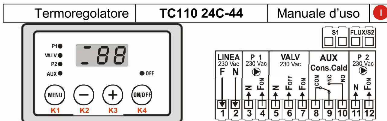
Fig. 1 Aspetto esterno e Schema dei collegamenti elettrici
